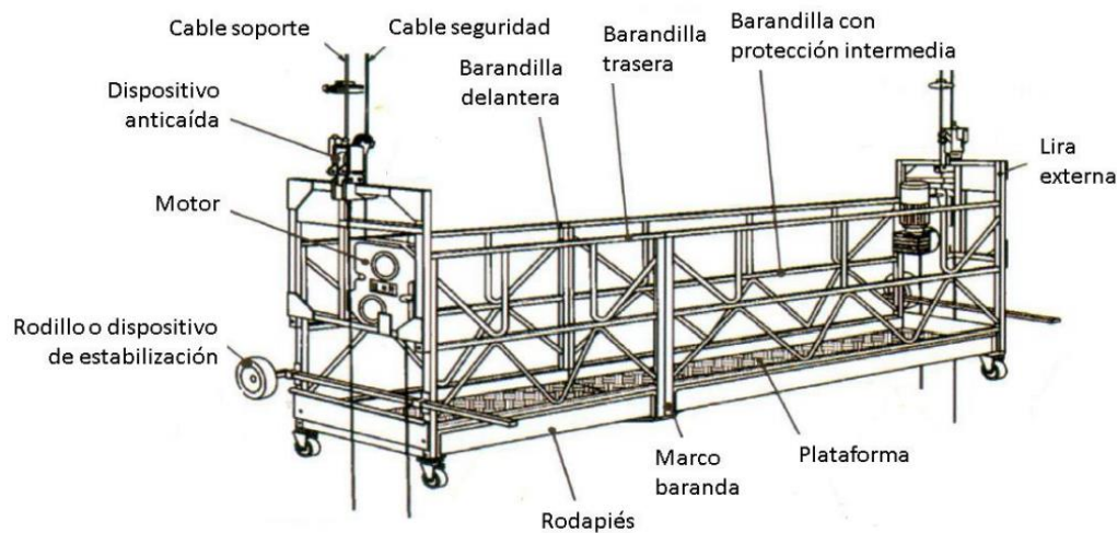
Figura 23. Andamios suspendidos.
